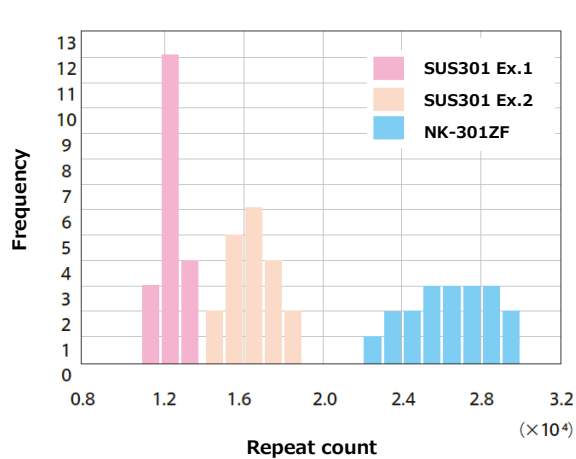
Fig.4 MIT test results
